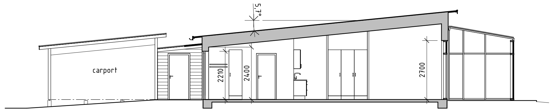
A2-A2 1:100
