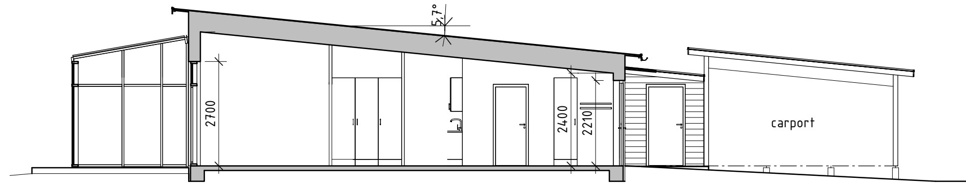
A1-A1 1:100
