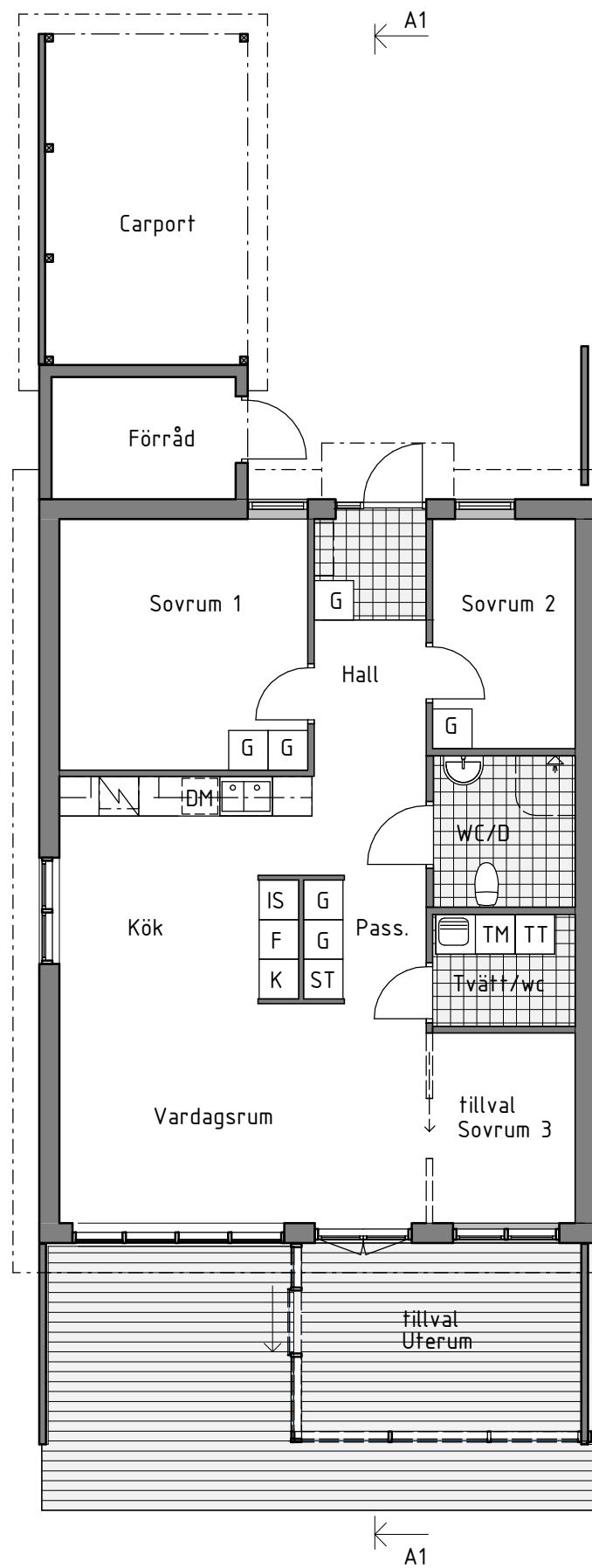
PLAN 1:100
