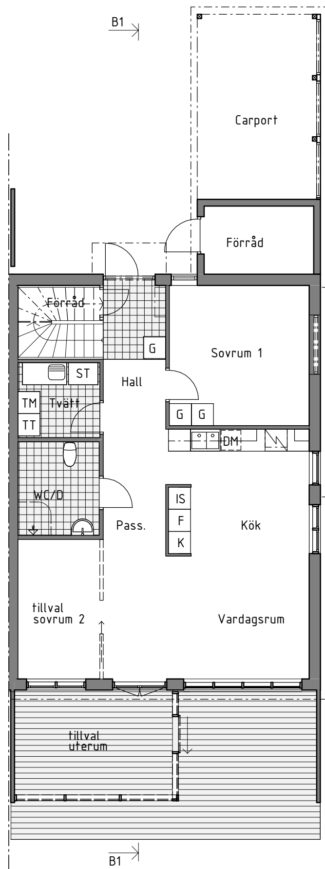
PLAN 1 1:100
