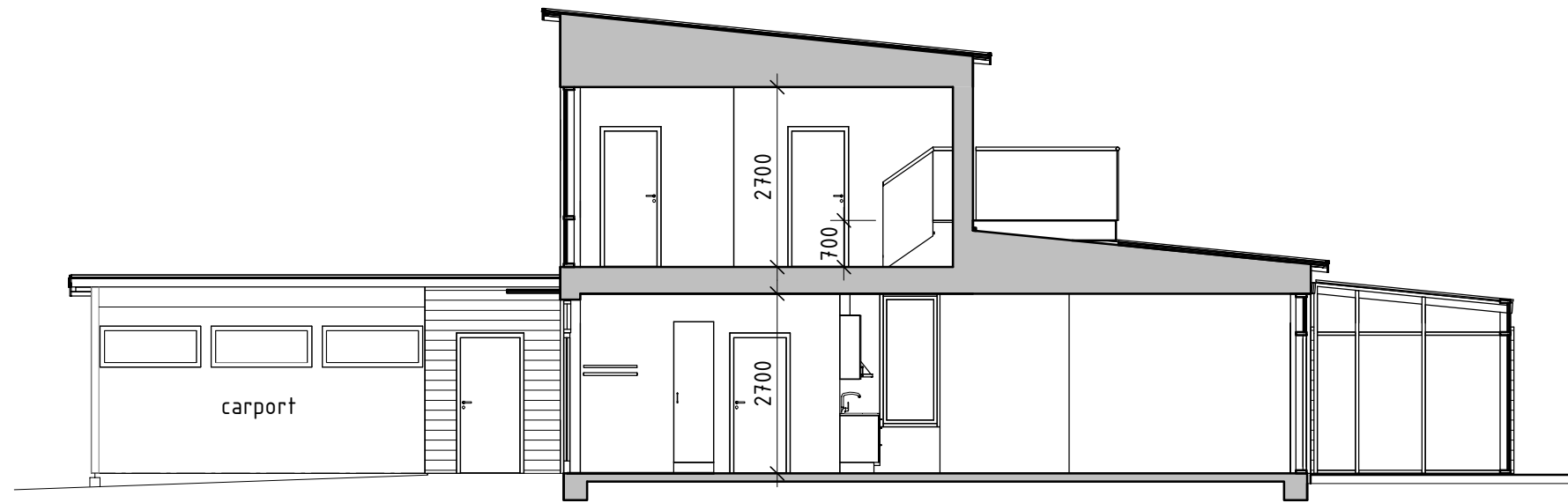
B1-B1 1:100
