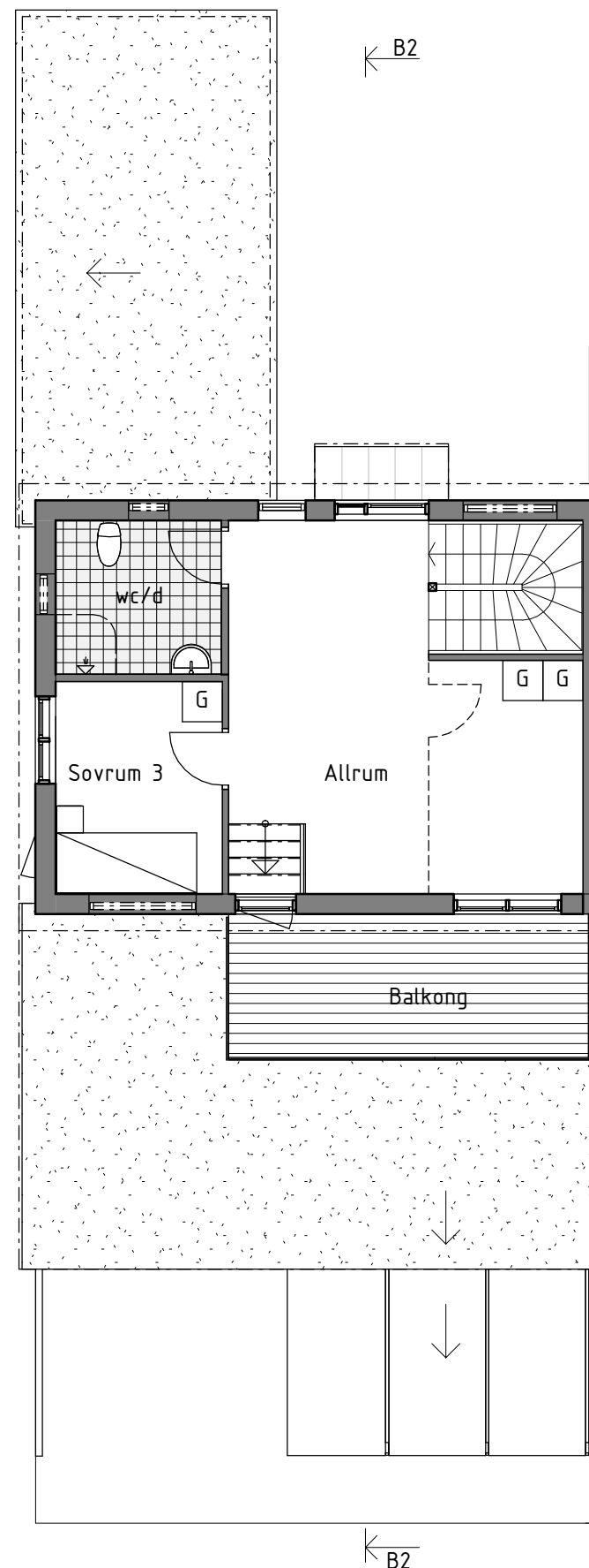
PLAN 2 1:100
