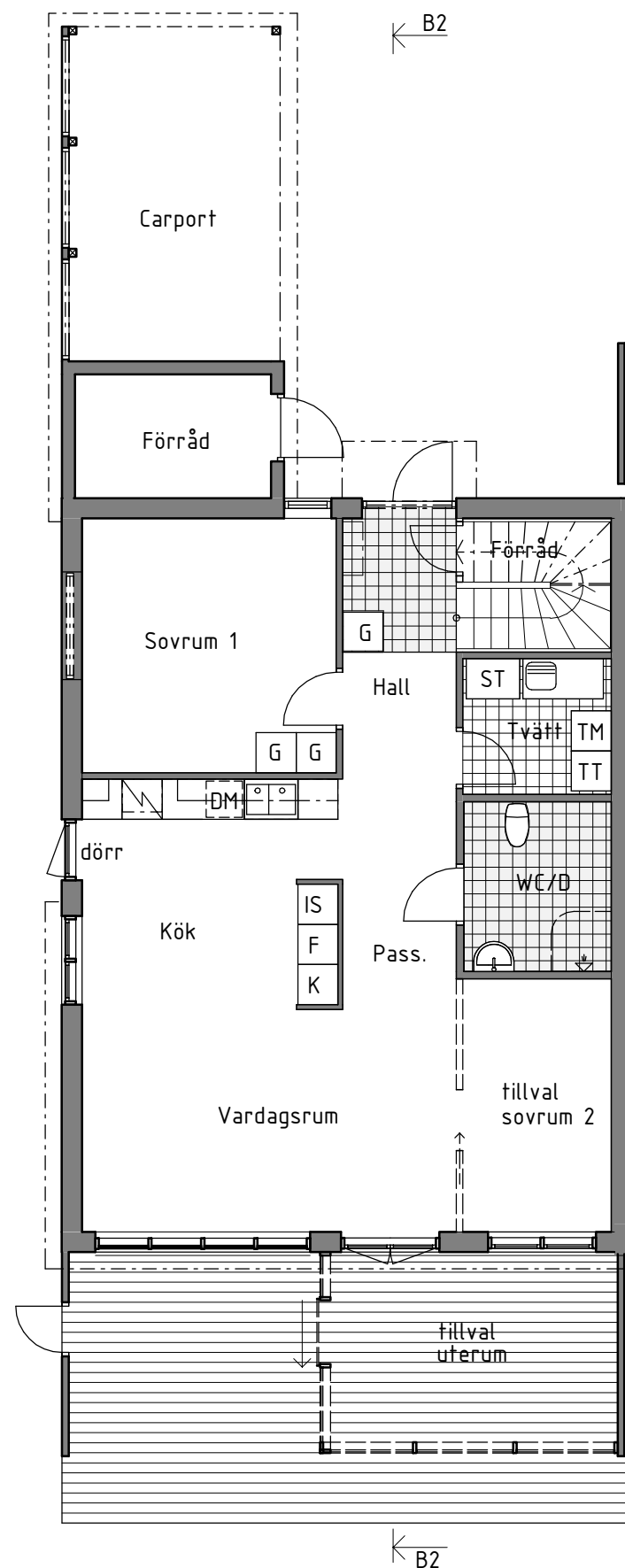
PLAN 1 1:100
